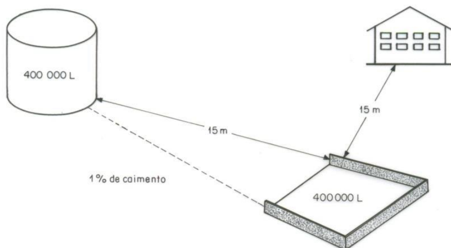
Figura 1.2: Bacia de contenção à distância.
