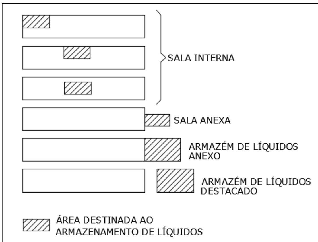
Figura 4.25: Exemplos das várias áreas internas de armazenamento de líquidos.
