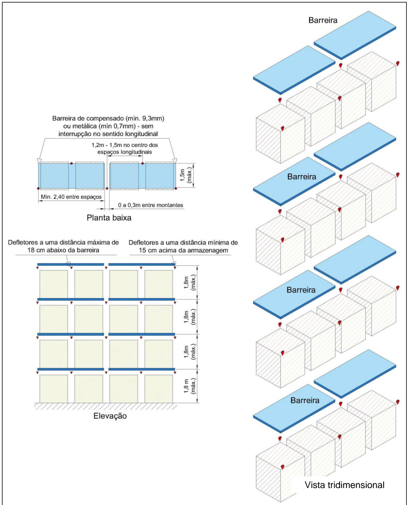
Figura 4.10: Leiaute de chuveiros automáticos para estrutura-suporte de fileira única – Esquema de projeto “B” – Chuveiros voltados para a estrutura. ( ▼ Chuveiros automáticos de níveis intermediários, chuveiros-spray, resposta rápida (QR), K=115. )
