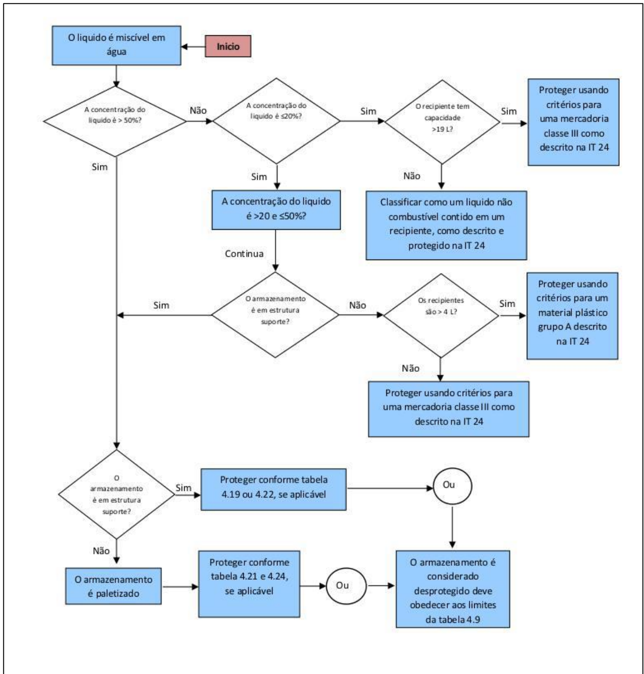
Figura 4.4: Árvore de decisão para o critério de proteção contra incêndio para líquidos inflamáveis e combustíveis miscíveis em água contido em recipientes não metálicos.
