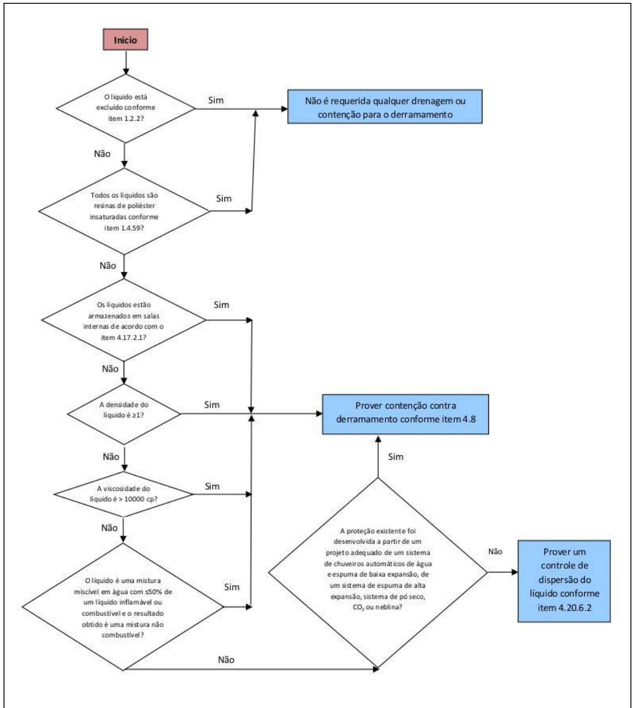
Figura 4.5: Contenção de derramamentos e controle de dispersão de líquidos em áreas de armazenamento protegido.
