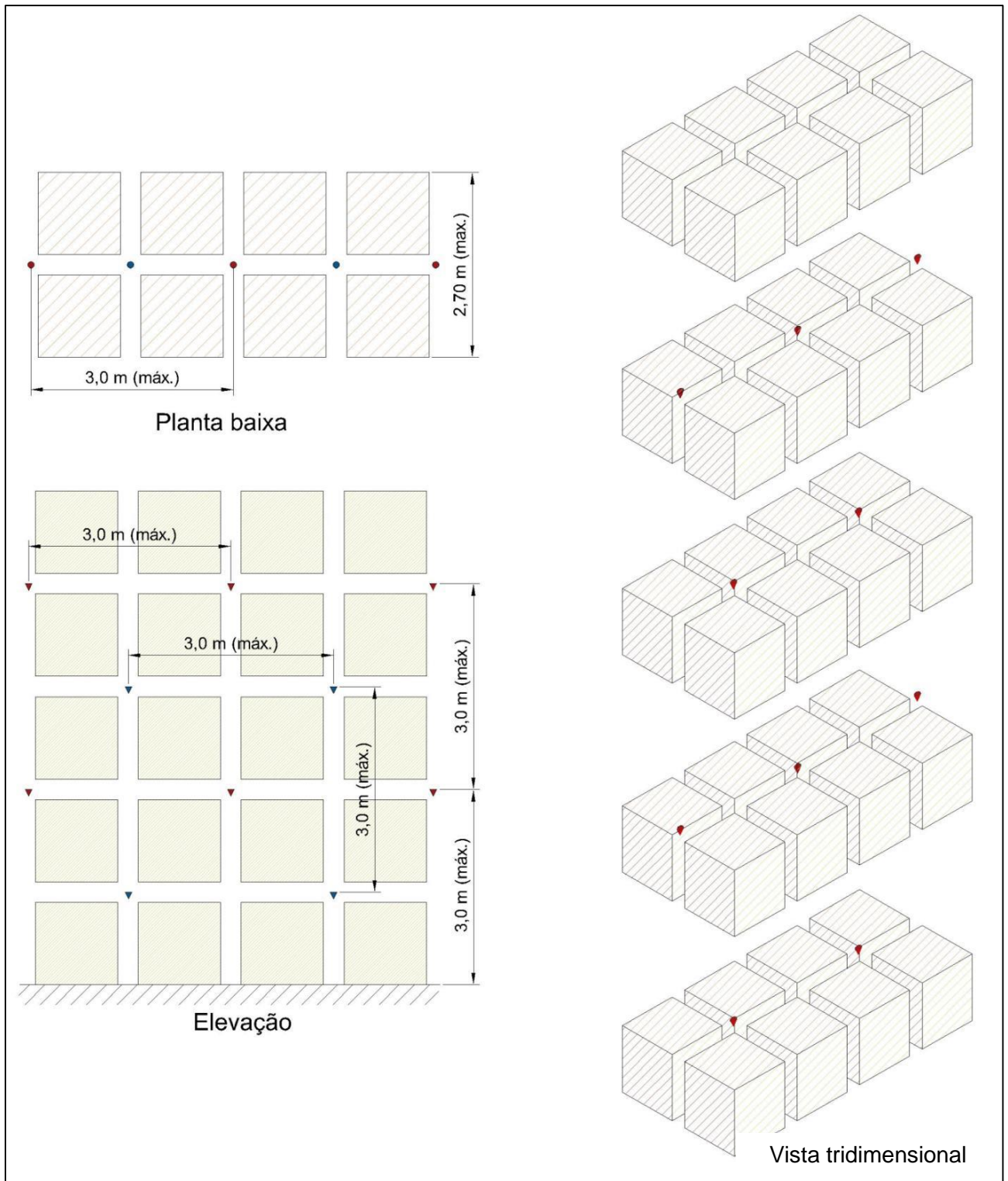
Figura 4.16: Leiaute de chuveiros automáticos para estrutura-suporte de fileira dupla – Leiaute “I”- Opção # 1. ( ▼ e ▼ Chuveiros automáticos de níveis intermediários, chuveiros-spray, resposta rápida (QR), K=115.)
