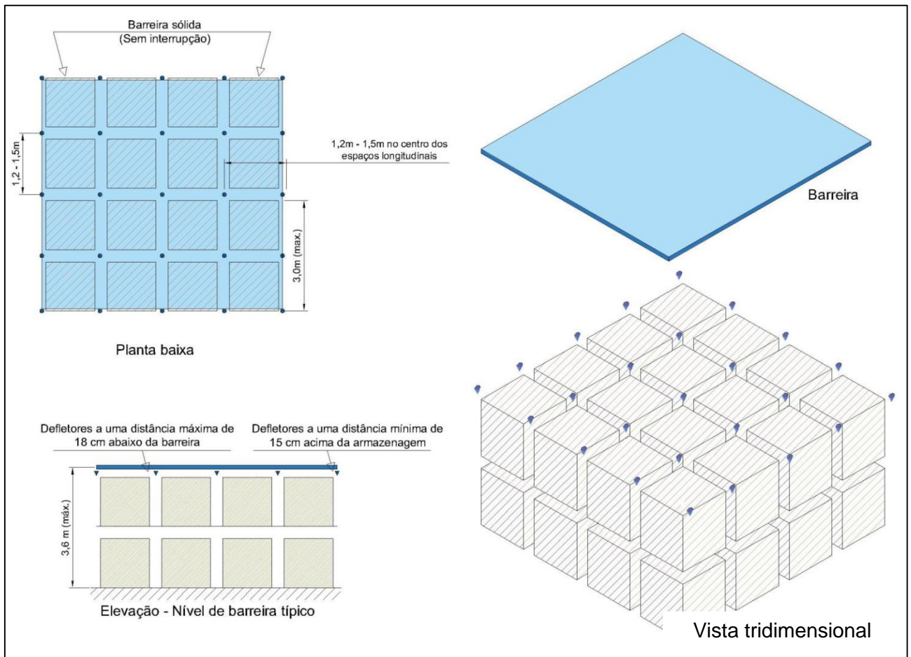
Figura 4.8: Leiaute de chuveiros automáticos para uma estrutura-suporte de múltiplas fileiras – Esquema de projeto “A”.
