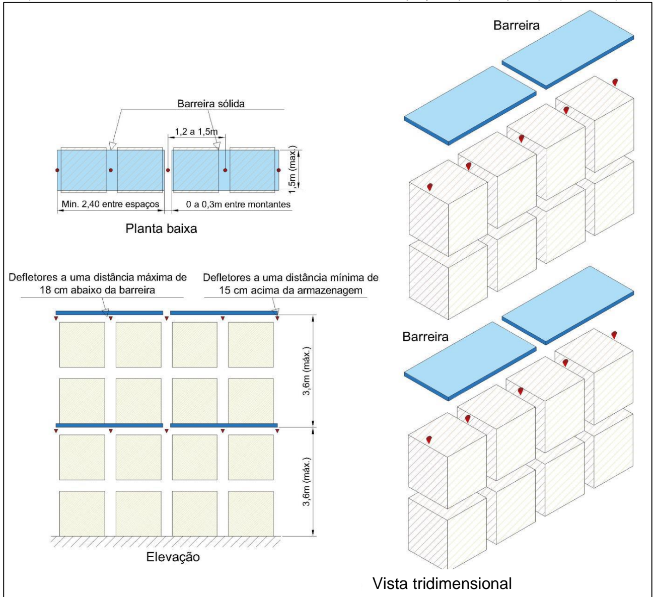
Figura 4.6: Leiaute de chuveiros automáticos para uma estrutura-suporte de fileira única Esquema de projeto “A”.
