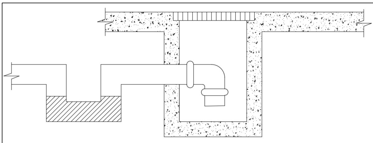
Figura 4.24: Detalhes de purgador selado por líquido.
