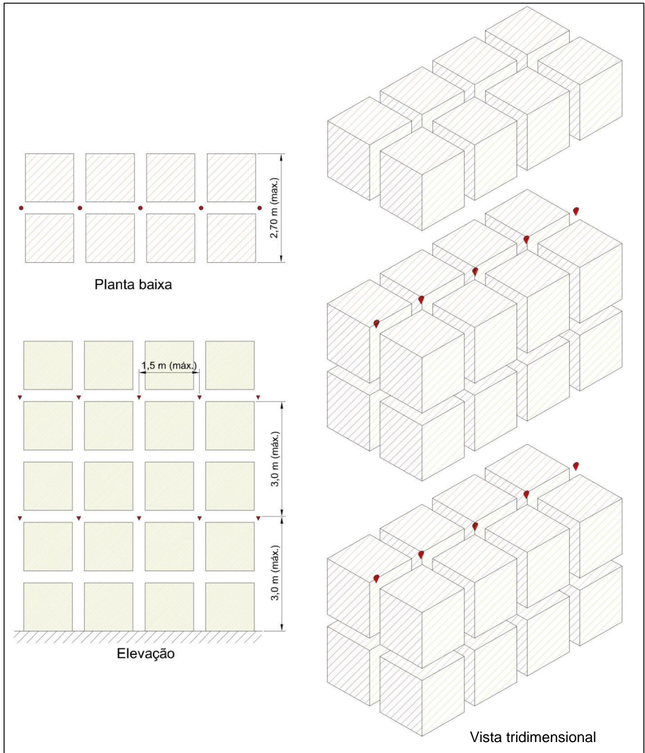
Figura 4.17: Leiaute de chuveiros automáticos para estrutura-suporte de fileira dupla – Leiaute “I” - Opção # 2 (▼ Chuveiros automáticos de níveis intermediários, chuveiros-spray, resposta rápida (QR), K=115.)
