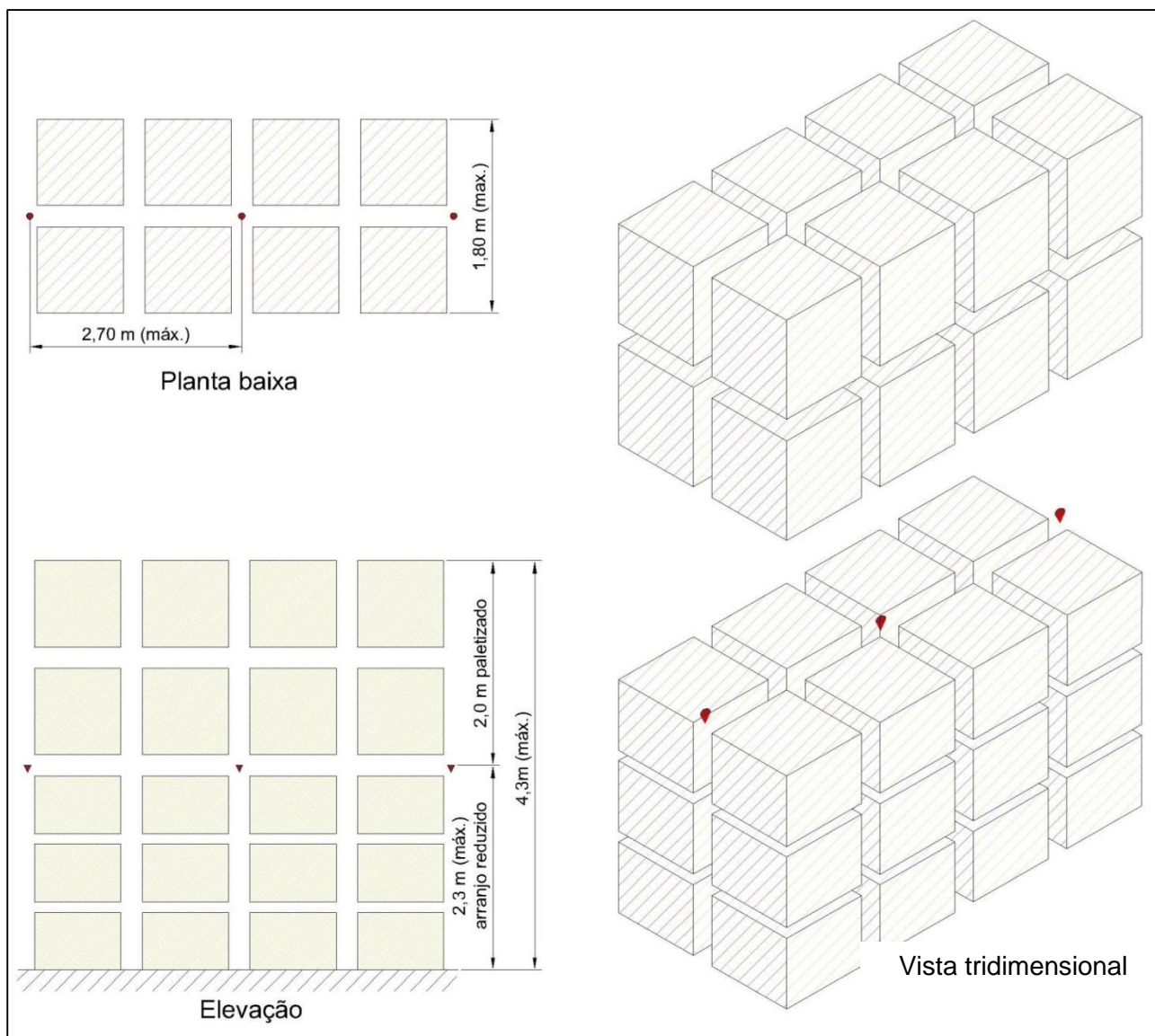
Figura 4.15: Leiaute de chuveiros automáticos para estrutura-suporte de fileira dupla – Leiaute "G". (▼ Chuveiros automáticos de níveis intermediários, chuveiros-spray, resposta rápida (QR), K=161.)
