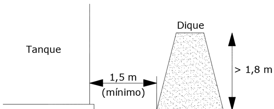
Figura 1.3: Distância mínima entre o costado do tanque e a base do dique.
