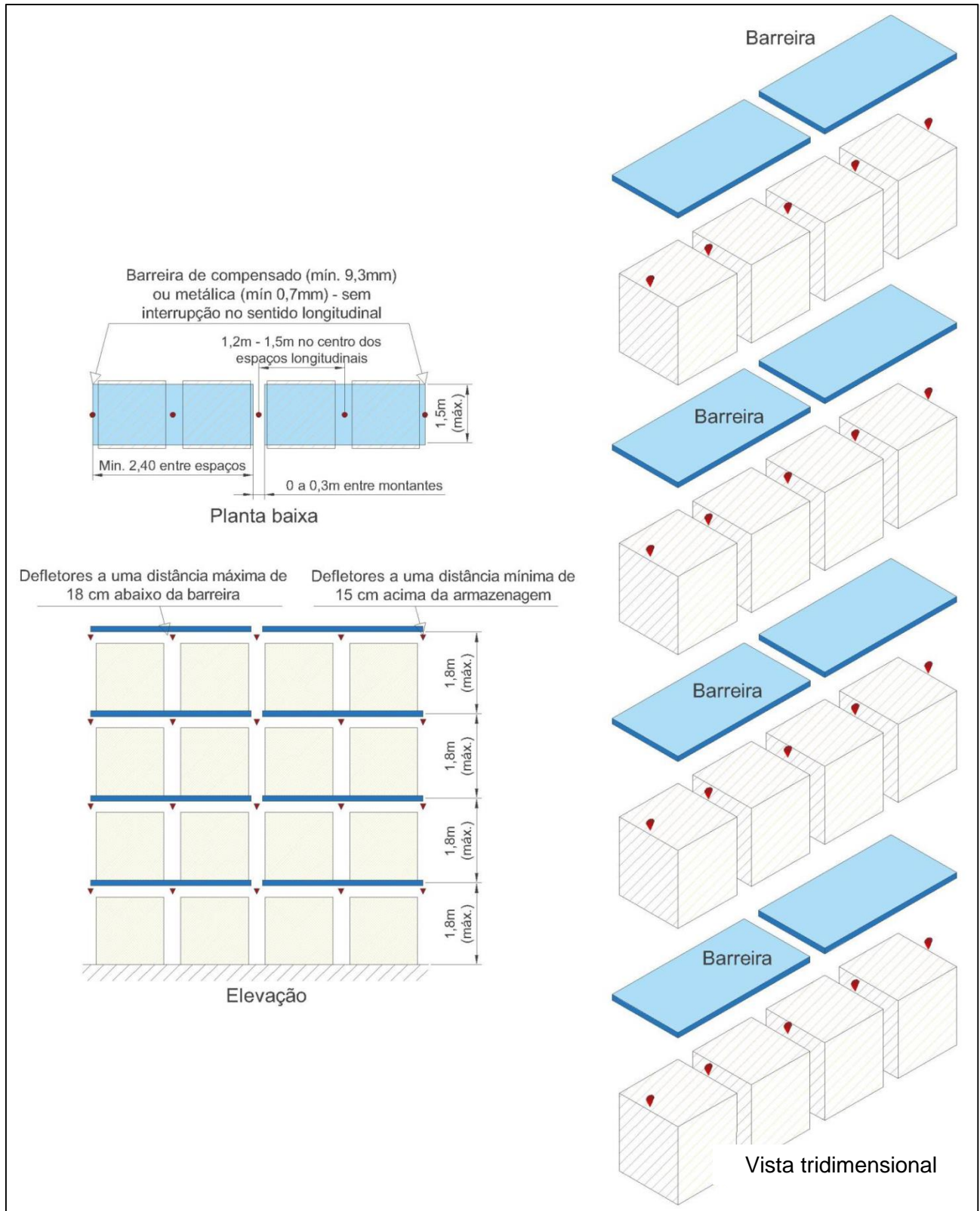
Figura 4.9: Leiaute de chuveiros automáticos para uma estrutura-suporte de fileira única Esquema de projeto “B” – Chuveiros no centro da estrutura (▼ Chuveiros automáticos de níveis intermediários, chuveiros-spray, resposta rápida (QR), K=115.)
