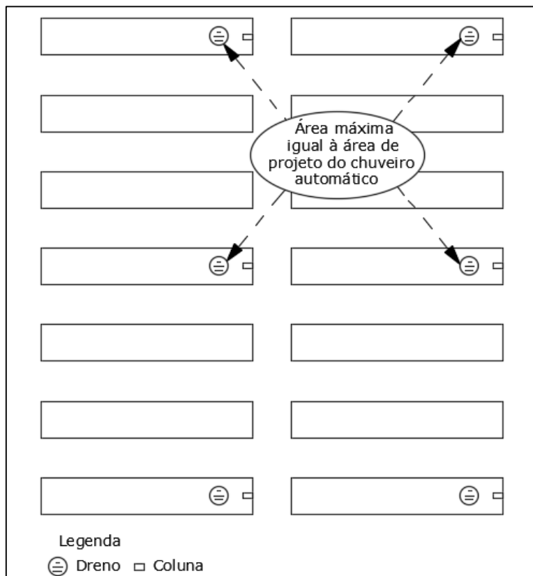
Figura 4.23: Arranjo típico de drenos de piso
