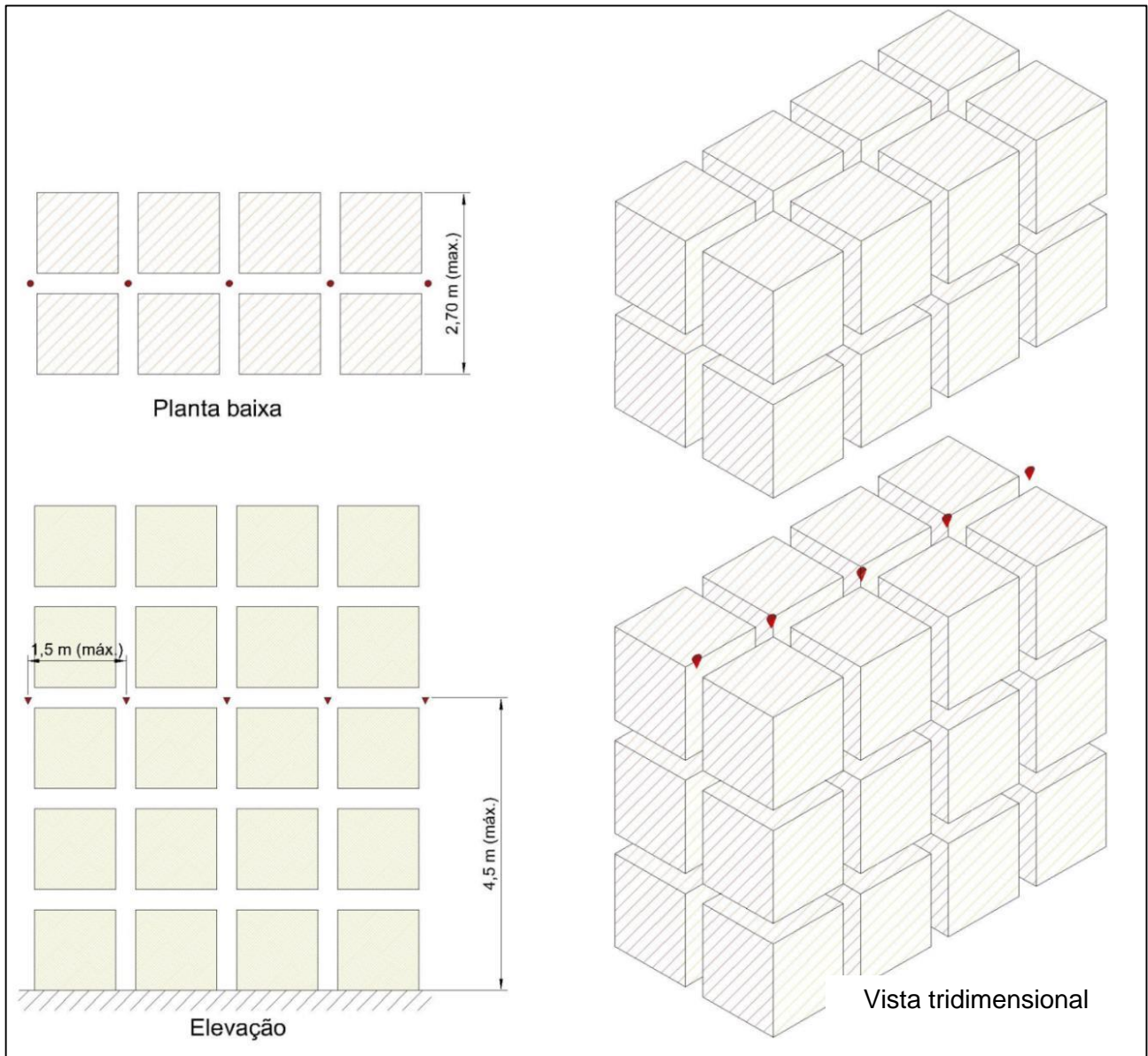
Figura 4.19: Leiaute de chuveiros automáticos para estrutura-suporte de fileira dupla – Leiaute “H” - Opção # 2. (▼ Chuveiros automáticos de níveis intermediários, chuveiros-spray, resposta rápida (QR), K=115.)
