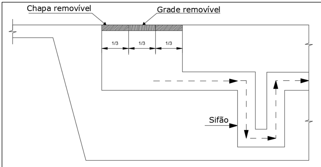
Figura 4.22: Detalhes do projeto de drenagem de canaletas.
