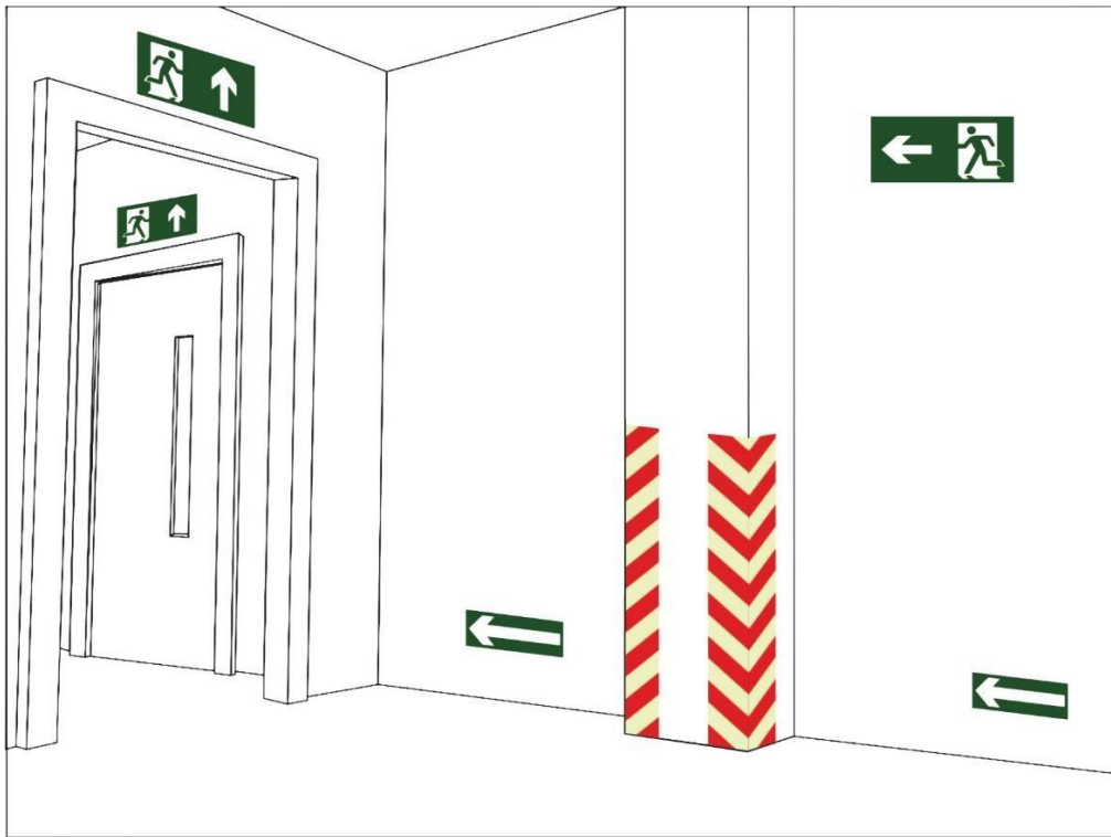
Figura C-9: Sinalização de saída sobre verga e portas, sinalização complementar de saídas e obstáculos.
