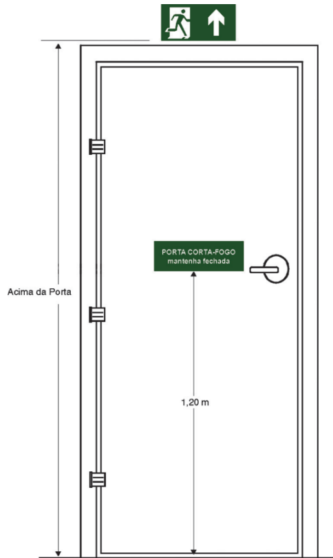
Figura C-1: Sinalização de porta corta-fogo (vista o hall)
