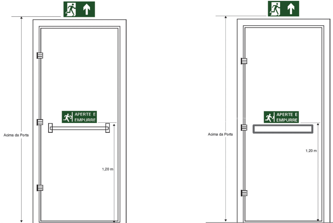
Figura C-5: Sinalização de portas com barra antipânico (modelos 1 e 2)
