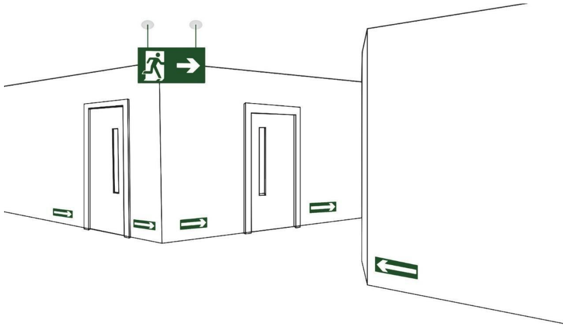
Figura C-13: Sinalização de saída perpendicular ao sentido da fuga, em dupla face.
