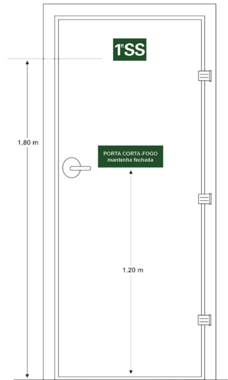
Figura C-2: Sinalização de porta corta-fogo (vista da escada)
