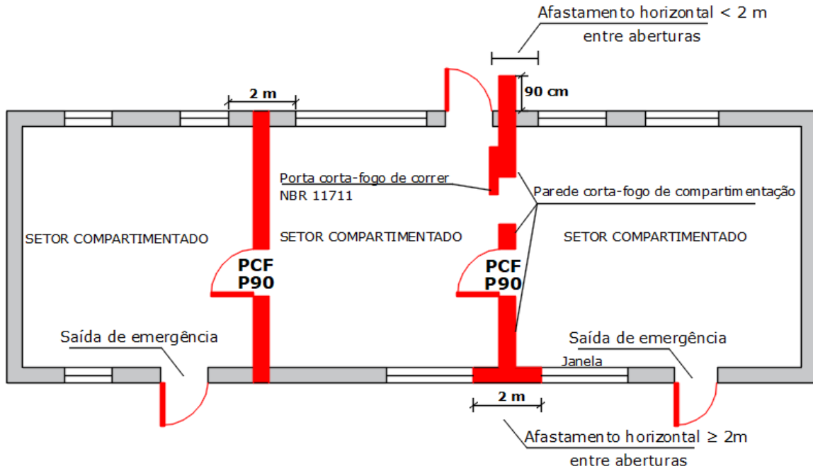
Figura A2: Modelo de compartimentação vertical (verga peitoril)
