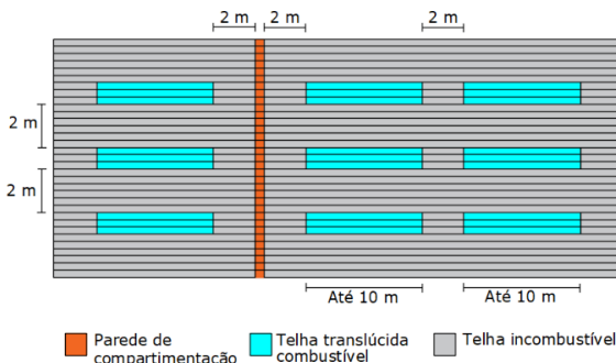
Figura 2: Afastamento de telhas translúcidas combustíveis.
