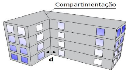
Figura 3: Fachadas ortogonais.
