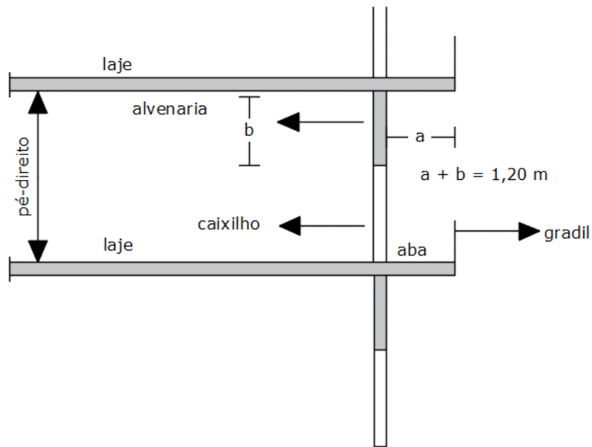
Figura A5: Modelo de compartimentação vertical (composição entre aba e verga-peitoril)
