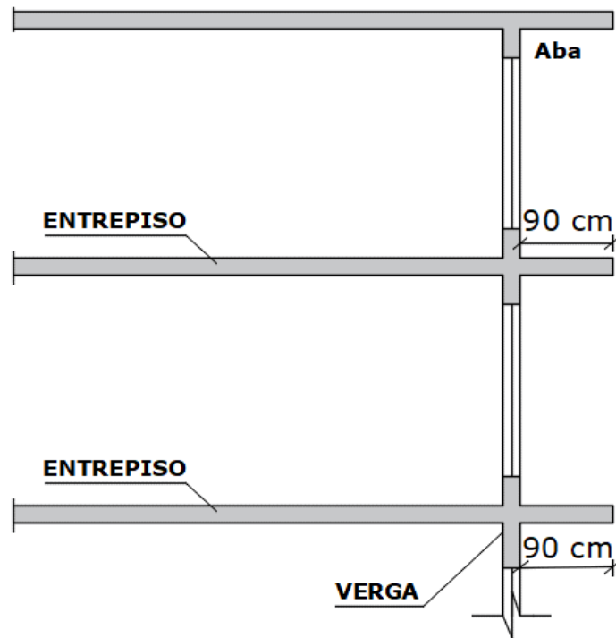
Figura A3: Modelo de compartimentação vertical (abas)
