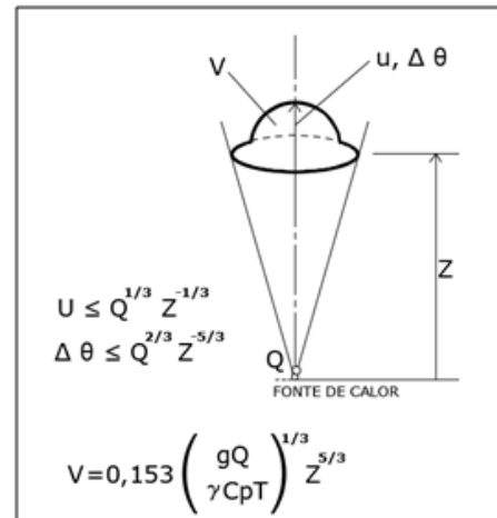
Figura 6: Plume de fumaça.
