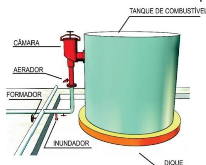
Figura 26 – Detalhe de câmara de espuma
