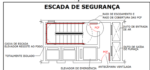
Figura 13: Escada e elevador à prova de fumaça.
