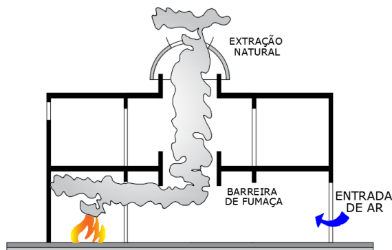
Figura 8: Extração de fumaça de átrios.
