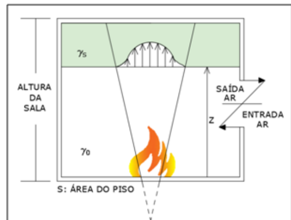
Figura 7: Processo de formação de gases e fluxo básico do ar.
