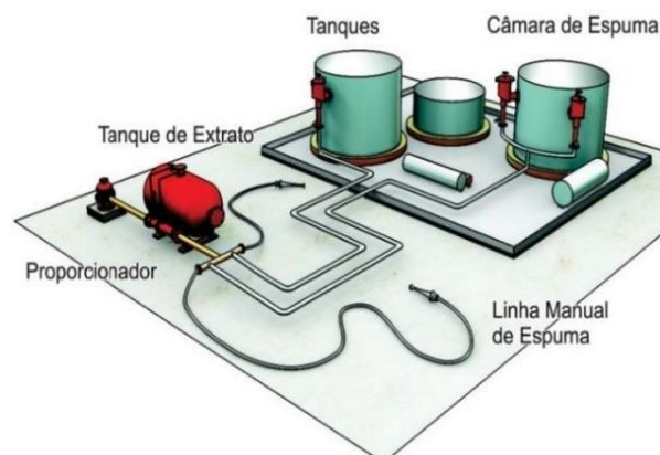
Figura 25 – Sistema semifixo
