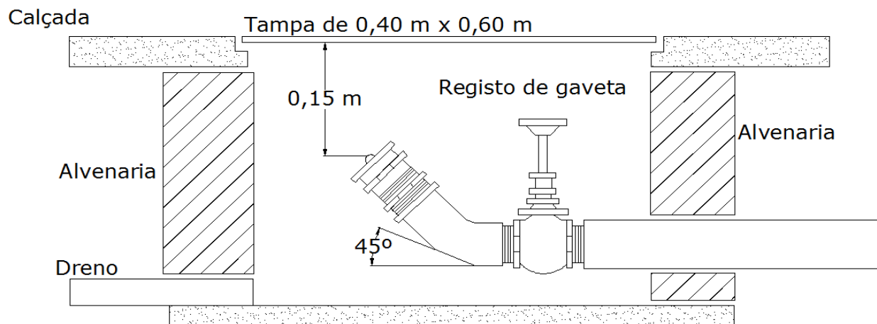
Figura 2 – Hidrante de recalque no passeio
