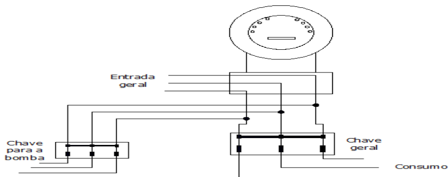
Figura 9 – Esquema de ligação elétrica da bomba de incêndio
